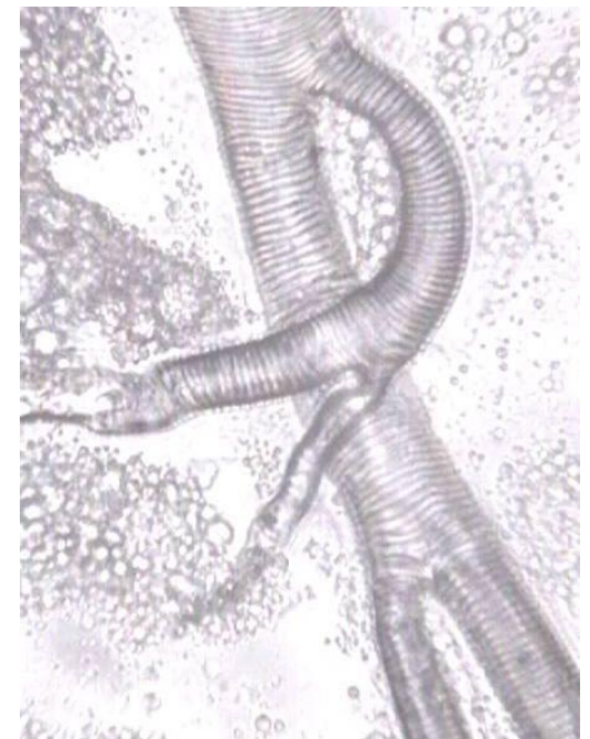
Trachée de Criquet
