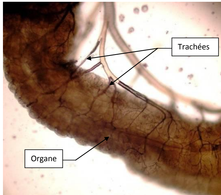
Trachée se ramifiant dans un organe
