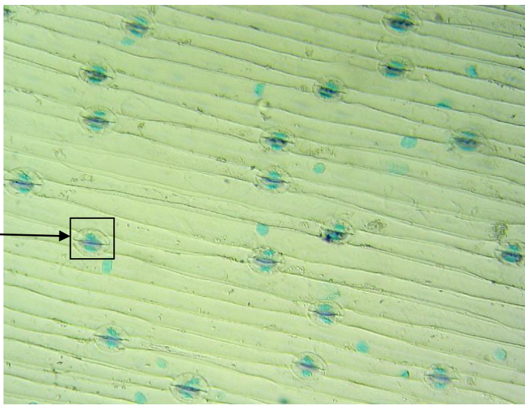
Stomates de Poireau
